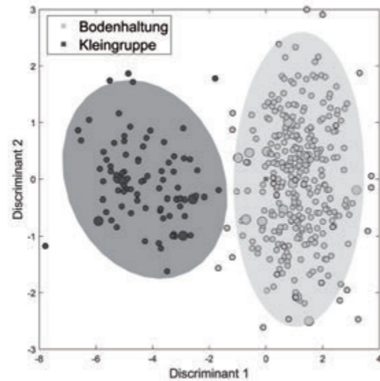
Abbildung 2: Lineare Diskriminanzanalyse (LDA) von den ^1\text{H-NMR} -Spektralen der Eigelbextraktproben aus Tabelle 3. Diese Proben stammen von Legehennen aus den zwei unterschiedlichen Haltungssystemen Bodenhaltung und Kleingruppenhaltung. Der LDA liegt eine Hauptkomponentenanalyse zur Dimensionsreduktion zu Grunde. Die LDA wurde mit einem Modell- und Testset gebildet. Das Testset besteht aus 20 zufällig ausgewählten Proben. Der unterlegte Bereich stellt das 95 %-Konfidenzintervall dar.
