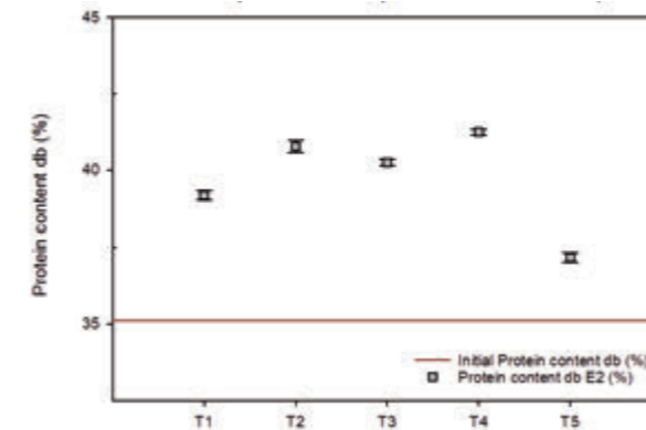
Proteingehalt im proteinangereicherten Fraktion nach triboelektrischer Trennung von kaltgepresstem Sonnenblumenmehl (20 % Öl)
