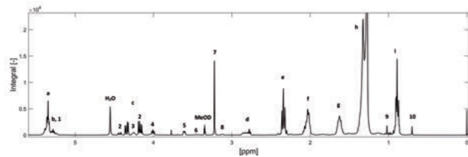
Abbildung 1: Darstellung des ^1\text{H-NMR} -Spektrums eines Eigelb-Extrakts in \text{CDCl}_3\text{-d}_1/\text{MeOD-d}_3 (3:2). Die Buchstaben a bis i bezeichnen die Signale im Spektrum, die mit Triacylglyceriden und ihren Fettsäuren (FS) zusammenhängen. b und c: Glycerol-Rückgrat, a: Vinyl-Wasserstoff, f: Allylic-methylen-Wasserstoff aller ungesättigter Fettsäuren, d: \text{CH}_2 -bis-allylic-Wasserstoff von PUFA ( \omega -3 und \omega -6 FS), e: Methylen-Gruppe an Carbonyl- \beta -Position, g: Methylen-Gruppe an Carbonyl- \alpha -Position, h: Ethyl-Gruppe, i: Methyl-Gruppe von FS. Die Nummern hängen mit den Signalen der Phospholipide und Cholesterol zusammen. Nummer 1, 2, 4 gehört zum Glycerol-Rückgrat, 3, 5, 7 zu Phosphatidylcholin, 4 und 8 zu Phosphatidylethanolamin und 6, 9, 10 zu Cholesterol. Signalzuordnung durch Ackermann et al. (2019).
